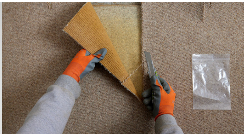
Prelievo di campioni da un vecchio rivestimento per pavimenti in materiale sintetico (ad es. sotto moquette): in caso di rivestimenti multistrato, occorre prelevare un campione che contenga tutti gli strati, colla compresa.
